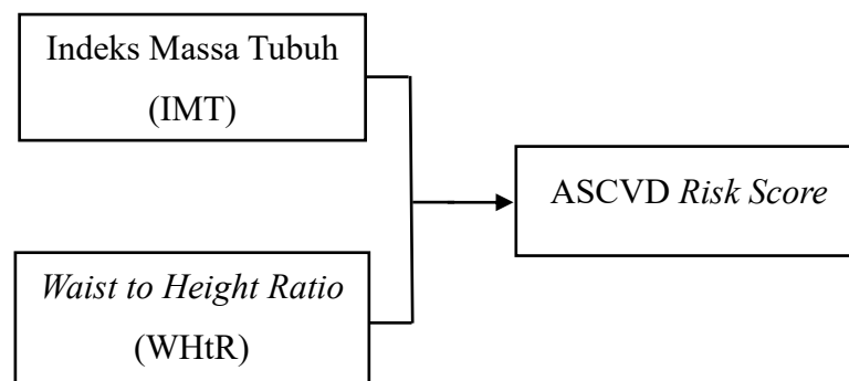
Gambar 3.2 Kerangka Konsep
