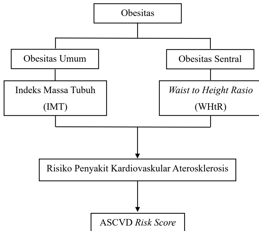
Gambar 3.1 Kerangka Teori
