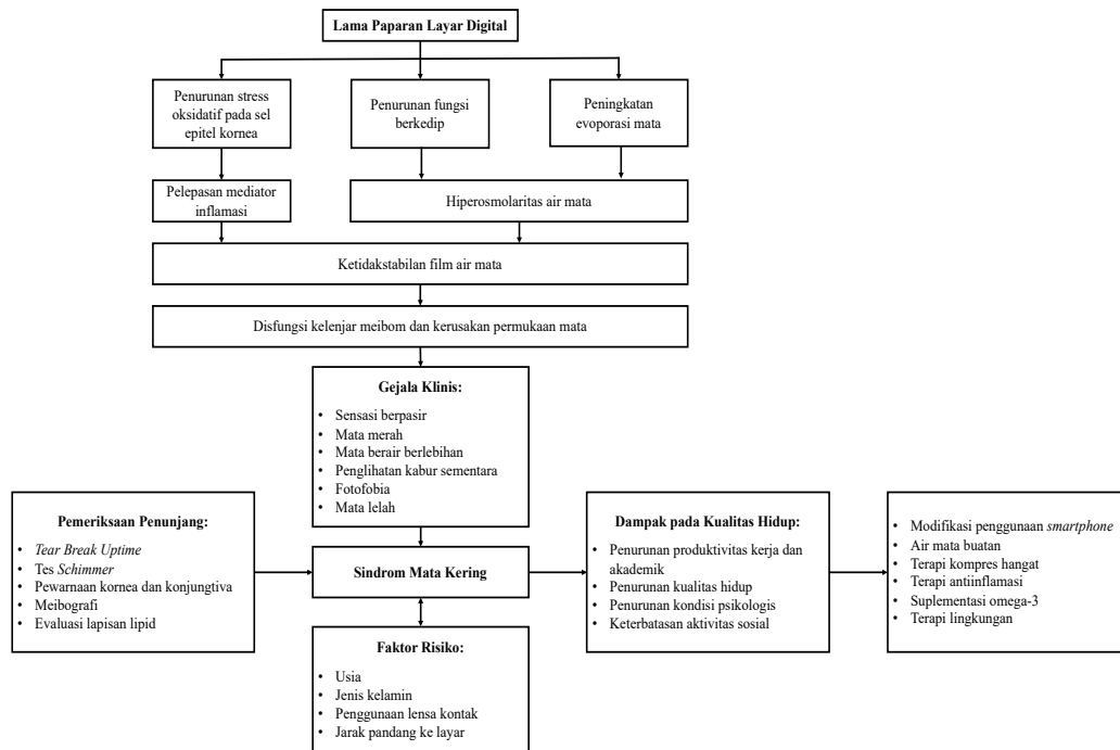
Gambar 3. 1 Kerangka Teori
