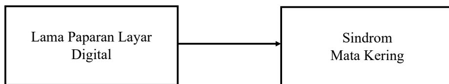
Gambar 3. 2 Kerangka Konsep
